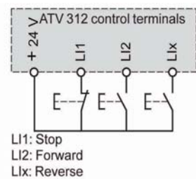
کنترل 3 سیمه
