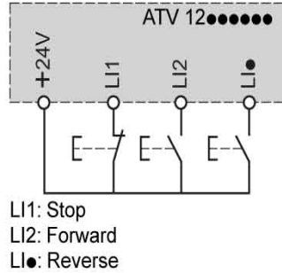
کنترل 3 سیمه
