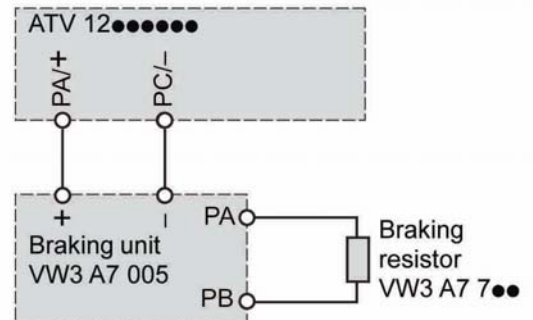
مقاومت ترمز
