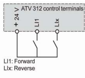
کنترل 2 سیمه
